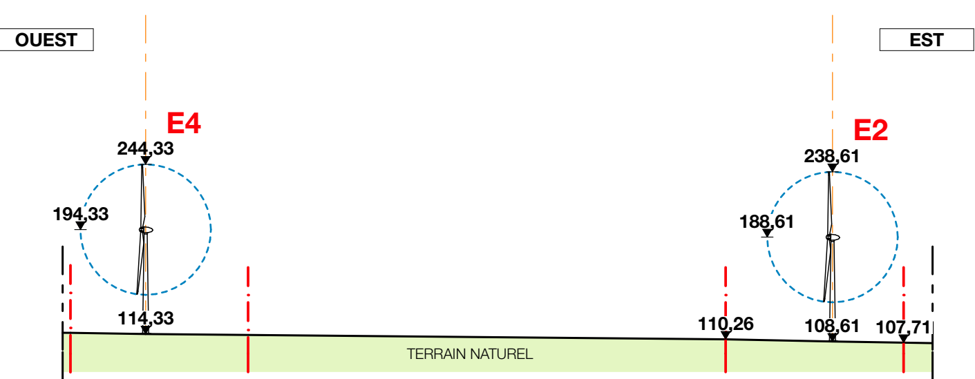
PROFIL SUD OUEST / NORD EST PROJET Ech. 1:4000
