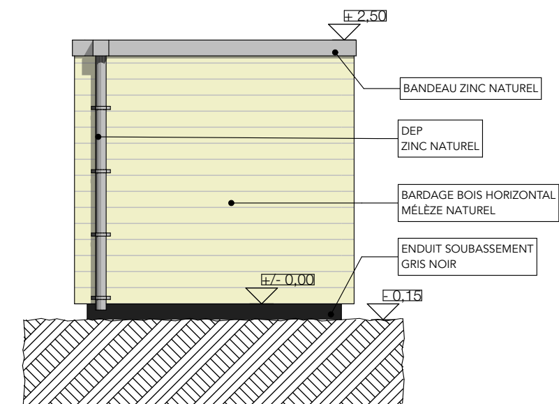
FAÇADE SUD Ech. 1:50
