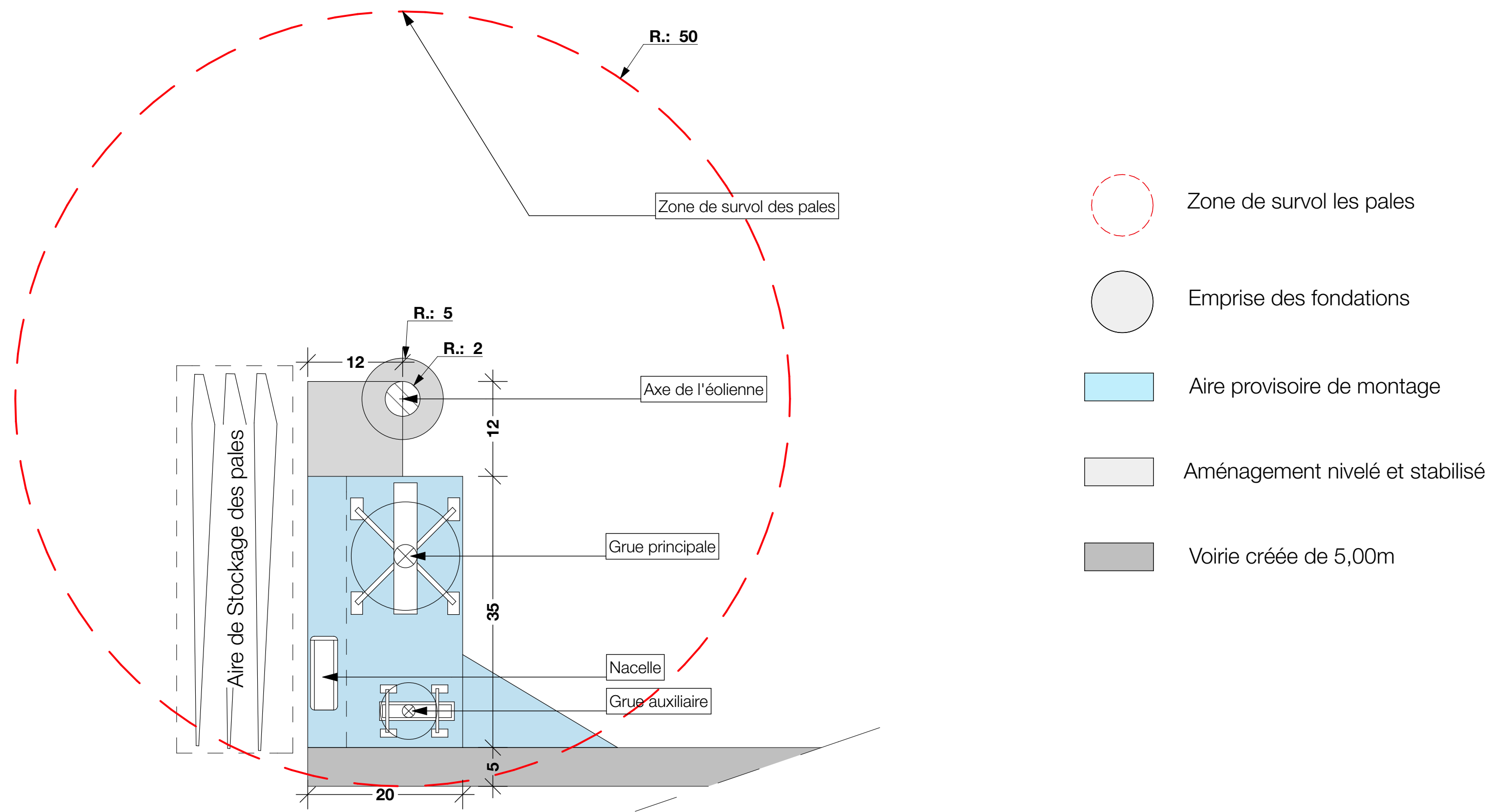
DÉTAIL D'UNE ÉOLIENNE PHASE TRAVAUX Ech. 1:500
