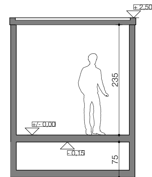
COUPE Ech. 1:50
