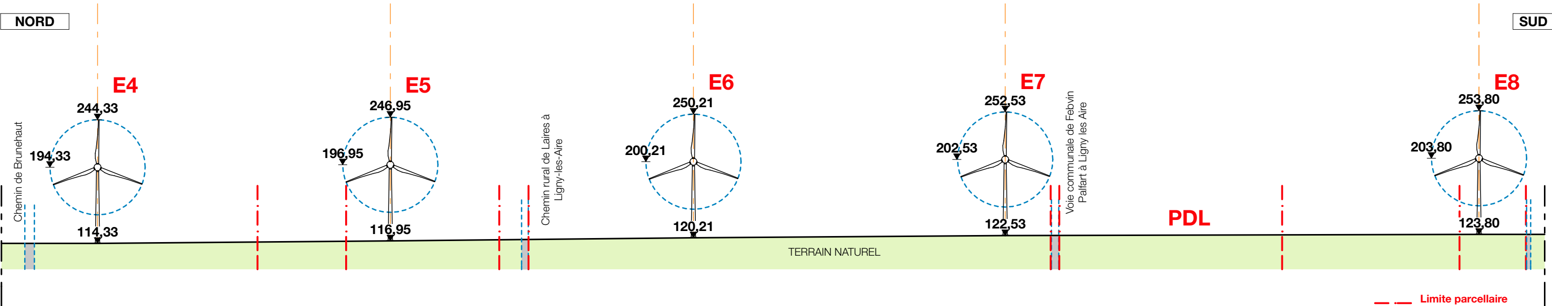
PROFIL NORD - OUEST / SUD - EST EXISTANT Ech. 1:4000
