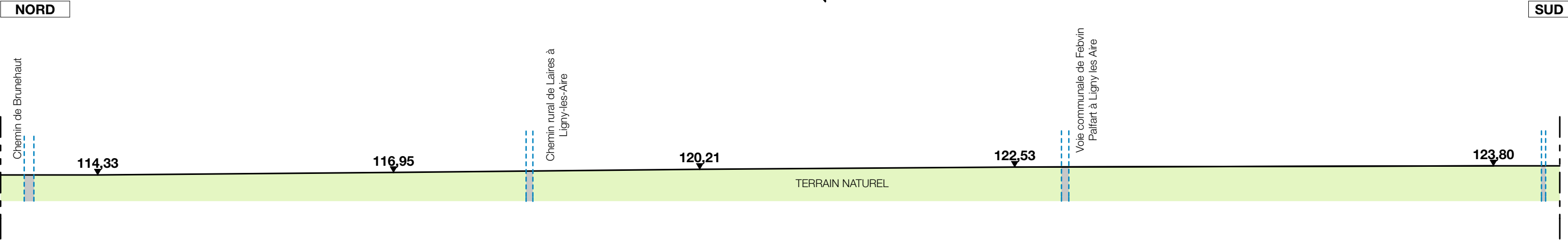
PROFIL NORD - OUEST / SUD - EST EXISTANT Ech. 1:4000
