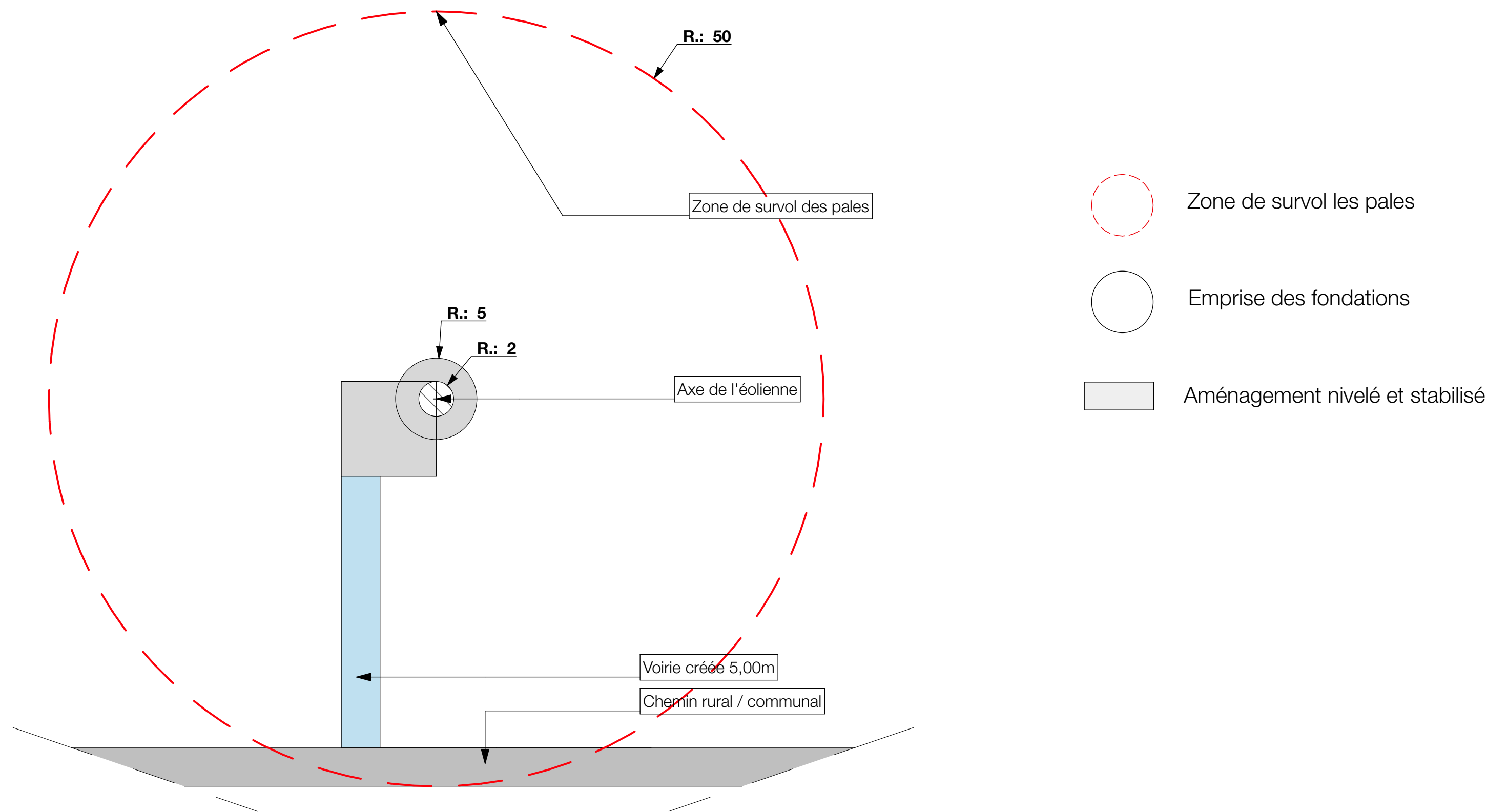
DÉTAIL D'UNE ÉOLIENNE PHASE EXPLOITATION Ech. 1:500
