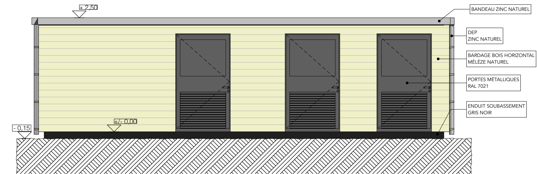
FAÇADE EST Ech. 1:50
