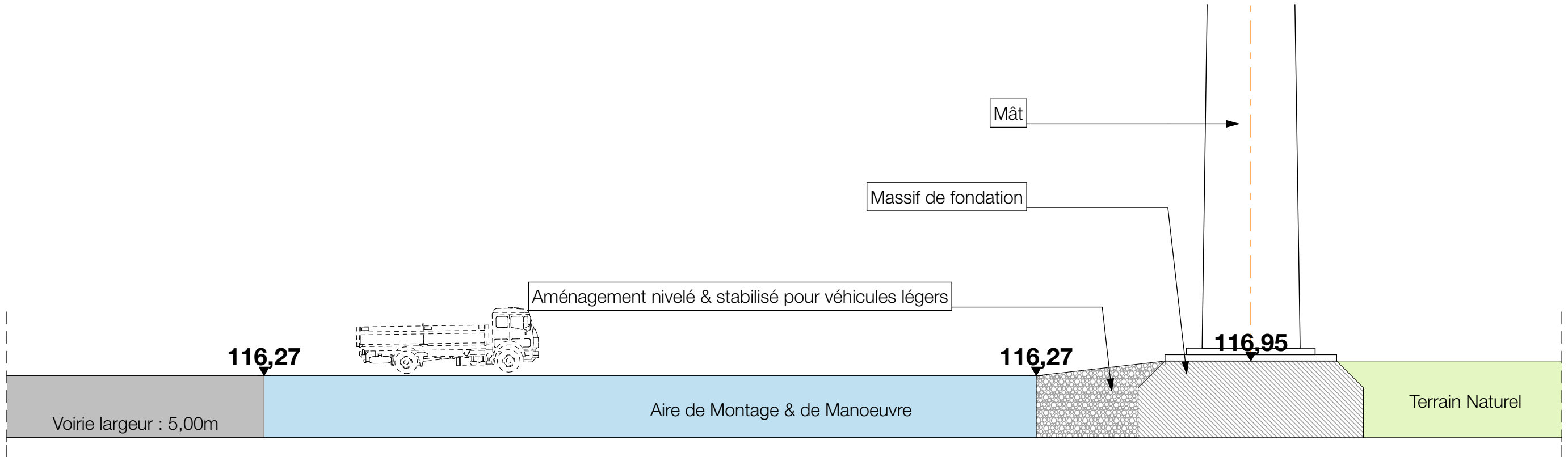
PROFIL ÉOLIENNE PROJET E5 Ech. 1:200
