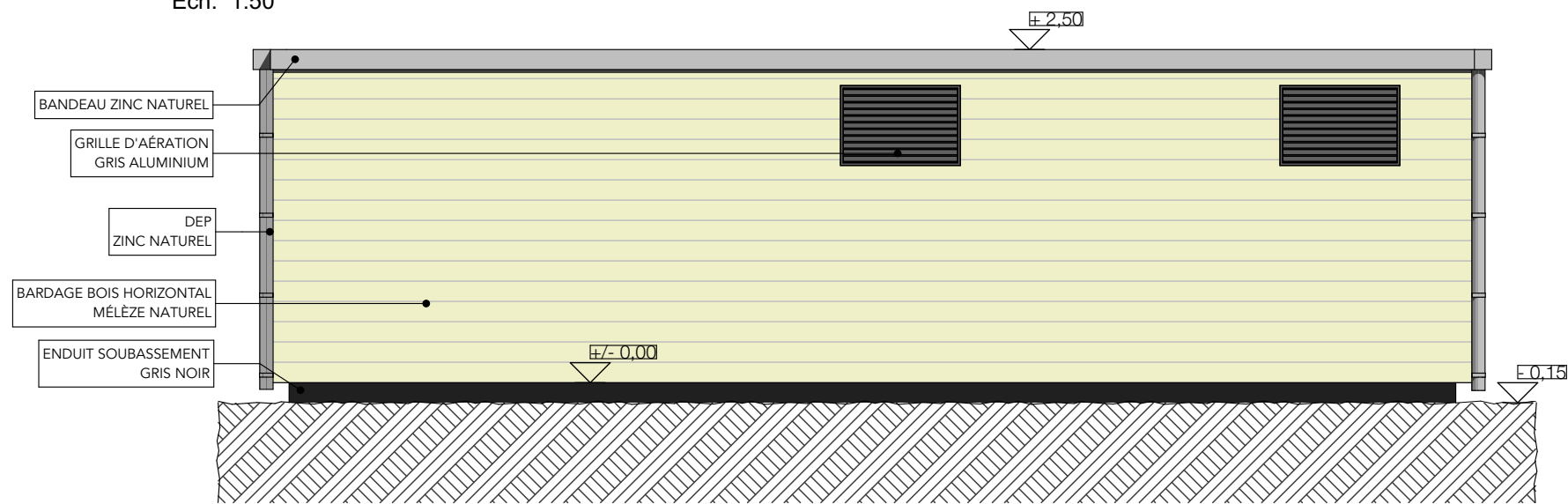
FAÇADE OUEST Ech. 1:50
