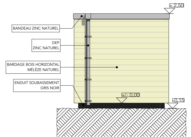
FAÇADE NORD Ech. 1:50
